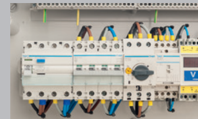
Amplio espacio para el cableado Wide space for the cabling
