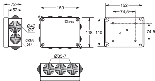
Caja con conos IP55 / Box with cones IP55 - Ref. Item 3032 4 72
