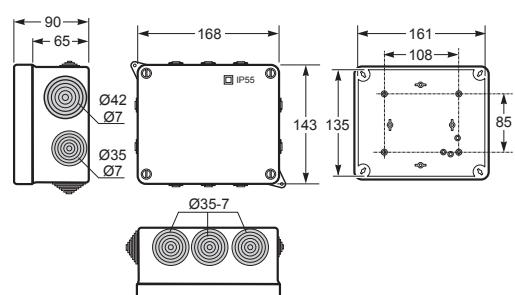
Caja con conos IP55 / Box with cones IP55 - Ref. Item 3033 1 42
