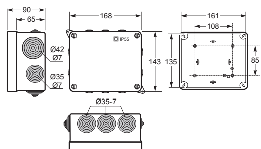
Caja con conos IP55 / Box with cones IP55 - Ref. Item 3013 1 42
